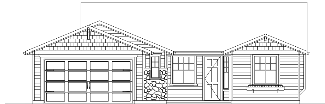
Elevation "C"
